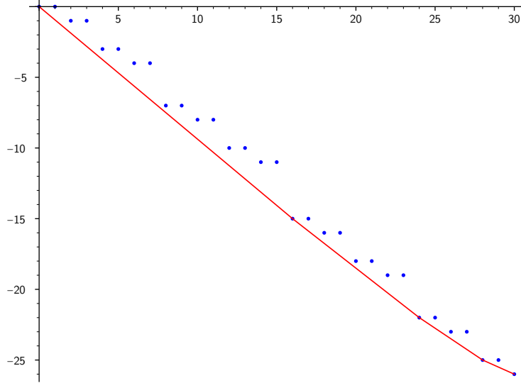
FIGURE 2. Polygone de Newton du polynôme \sum_{n=0}^{30} T^n/n! pour la valeur absolue 2-adique. Les 4 pentes correspondent à la décomposition 30 = 2^4 + 2^3 + 2^2 + 2
