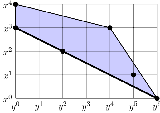
FIGURE 1. L'exemple de Newton : \varphi = y^6 - 5xy^5 + (x^3/a)y^4 - 7a^2x^2y^2 + 6a^3x^3 + b^2x^4 = 0
